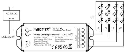
FUT044 A vezérlő csatlakoztatása az RGBW LED-szalaghoz
