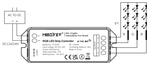
FUT043 A vezérlő csatlakoztatása az RGB LED-szalaghoz
