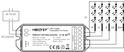
FUT045 A vezérlő csatlakoztatása az RGB+CCT LED-szalaghoz
